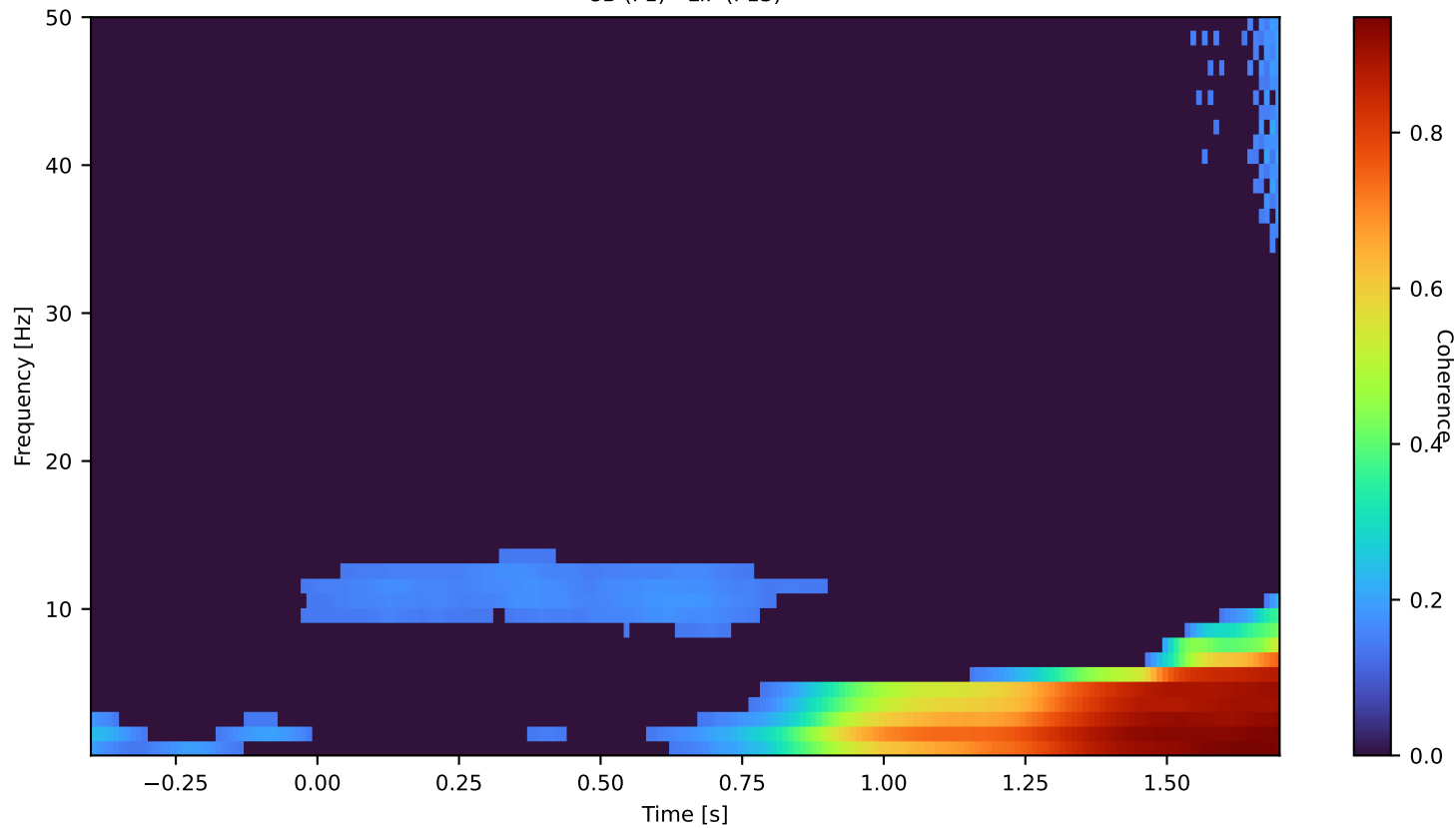
8B (F1) - LIP (P13)
